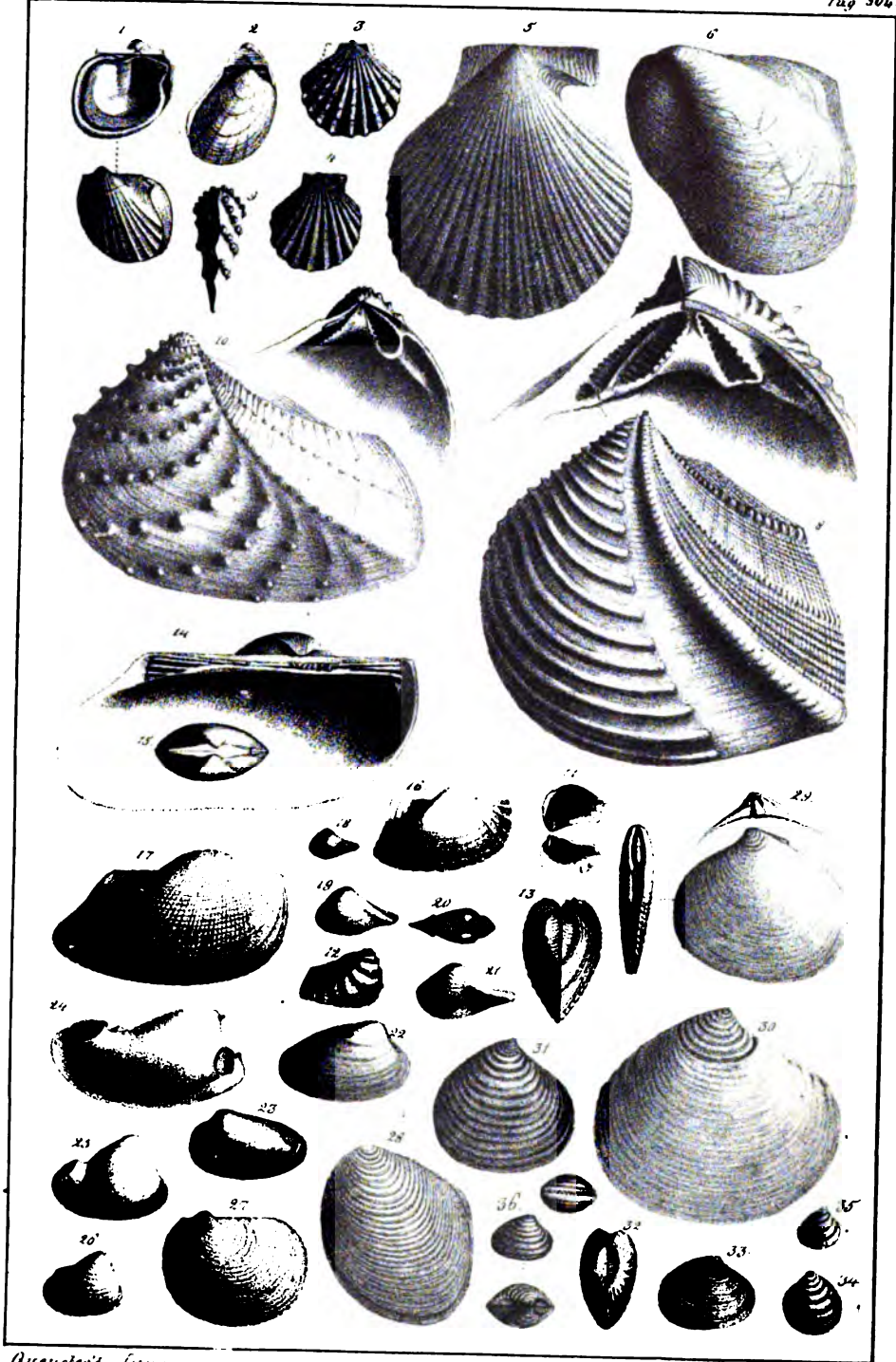
Quenstedt's Atlas
